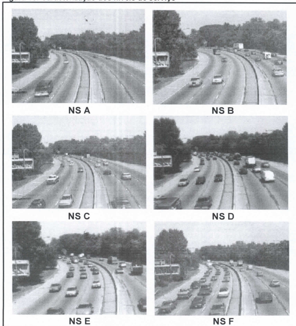
Figura 18: Caracterização dos níveis de serviço
