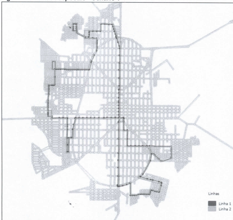
Figura 77: Linhas Propostas - Cenário 1
