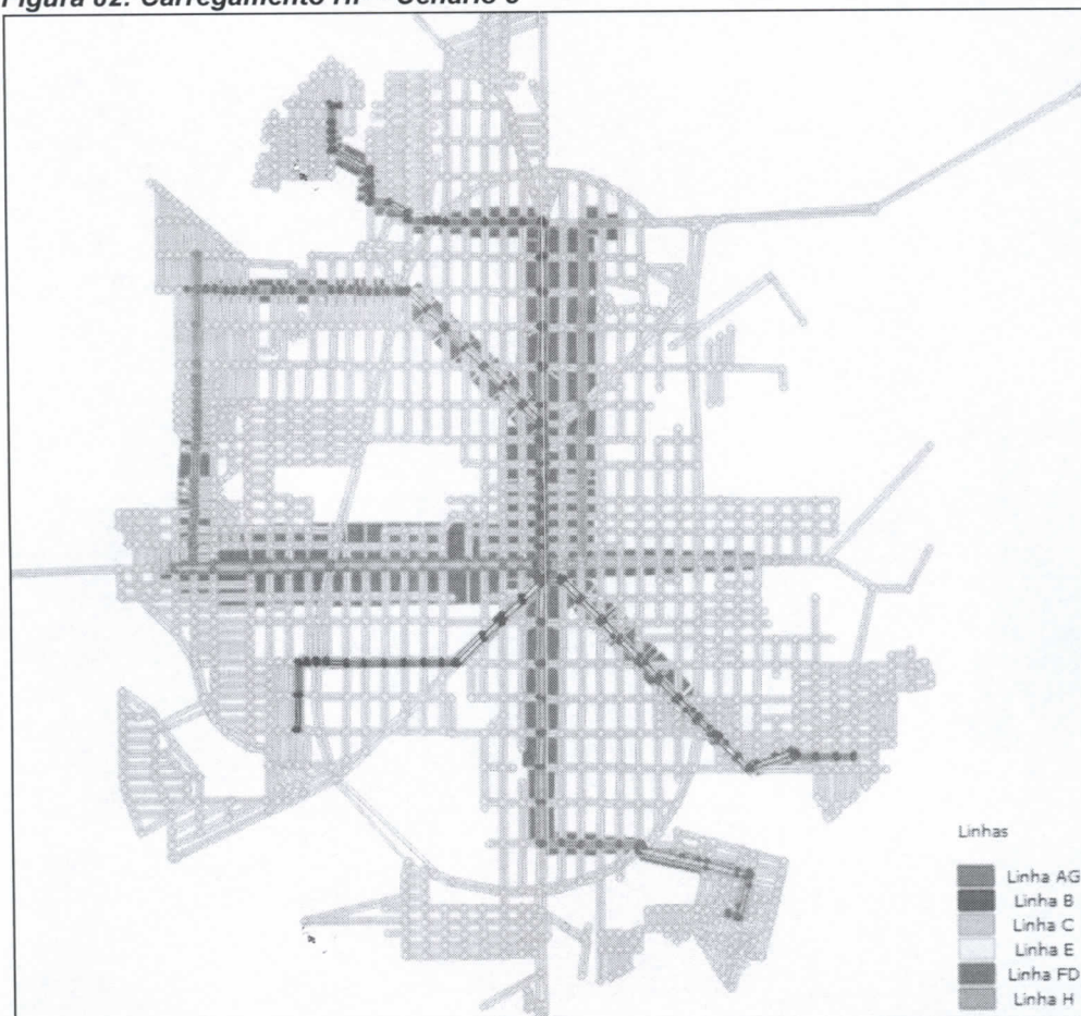
Figura 82: Carregamento HP - Cenário 3
