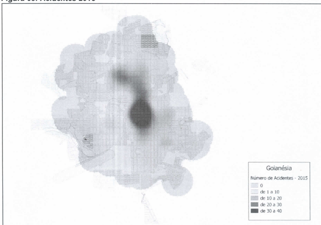
Figura 68: Acidentes 2015
