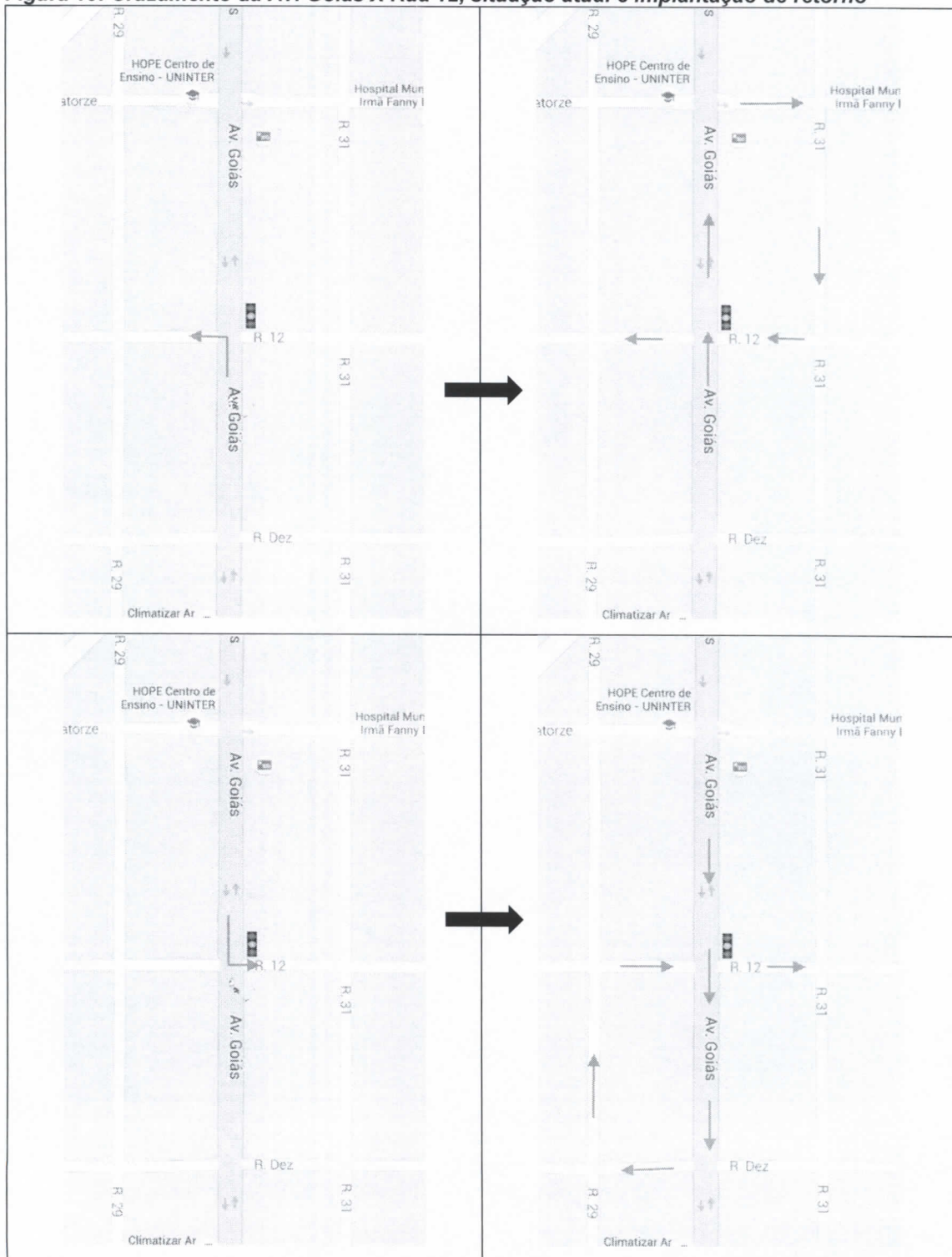
Figura 19: Cruzamento da Av. Goiás X Rua 12, situação atual e implantação de retorno
